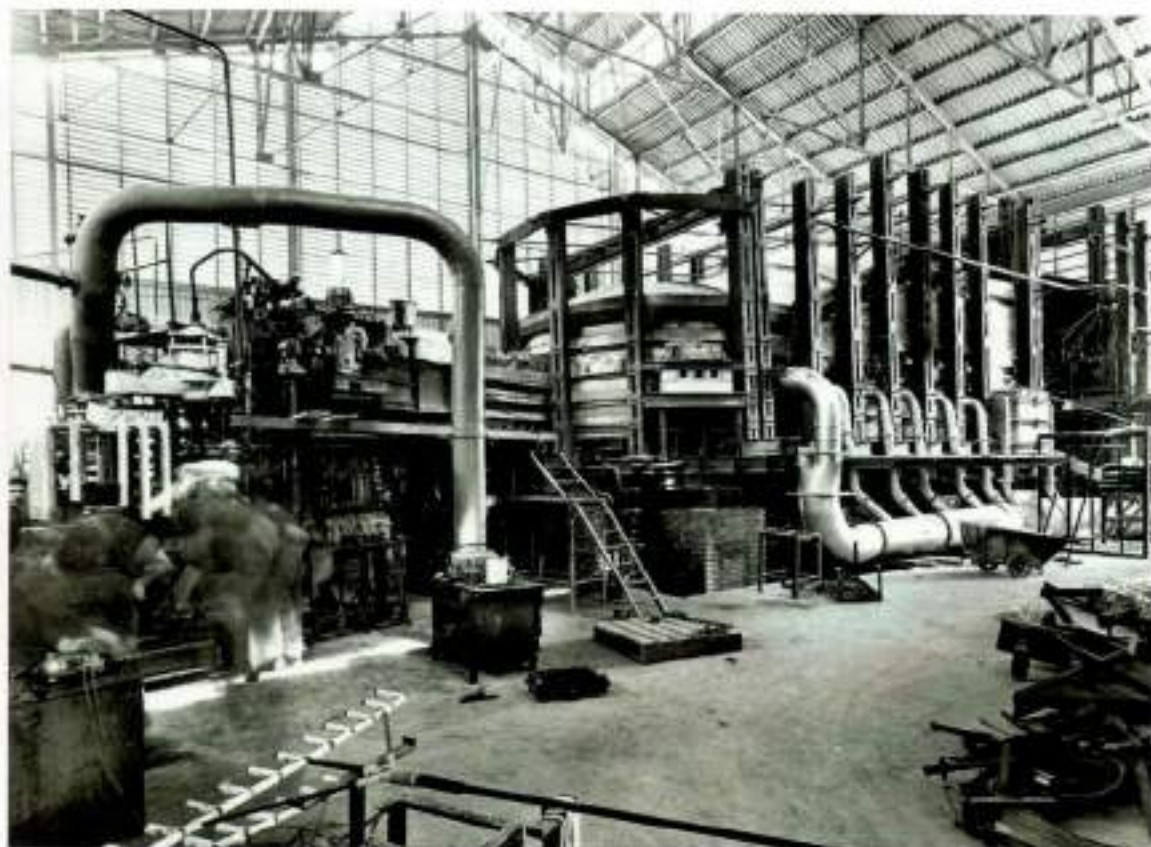
Forn núm. 5, feeder i premsa. ELSA, S.A. Fons Sans. AHMC.
