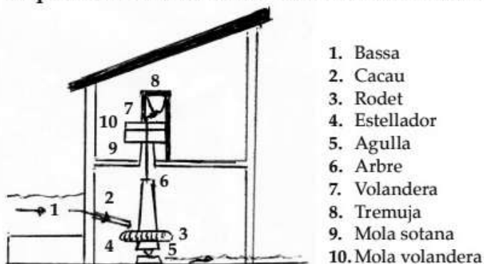
Esquema de funcionament d'un molí hidràulic
